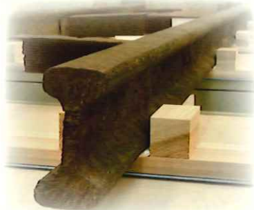
汐留駅の側線に使用されていた双頭レール 物流博物館蔵
